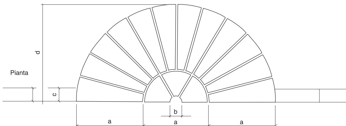
Schema "Ventaglio"
